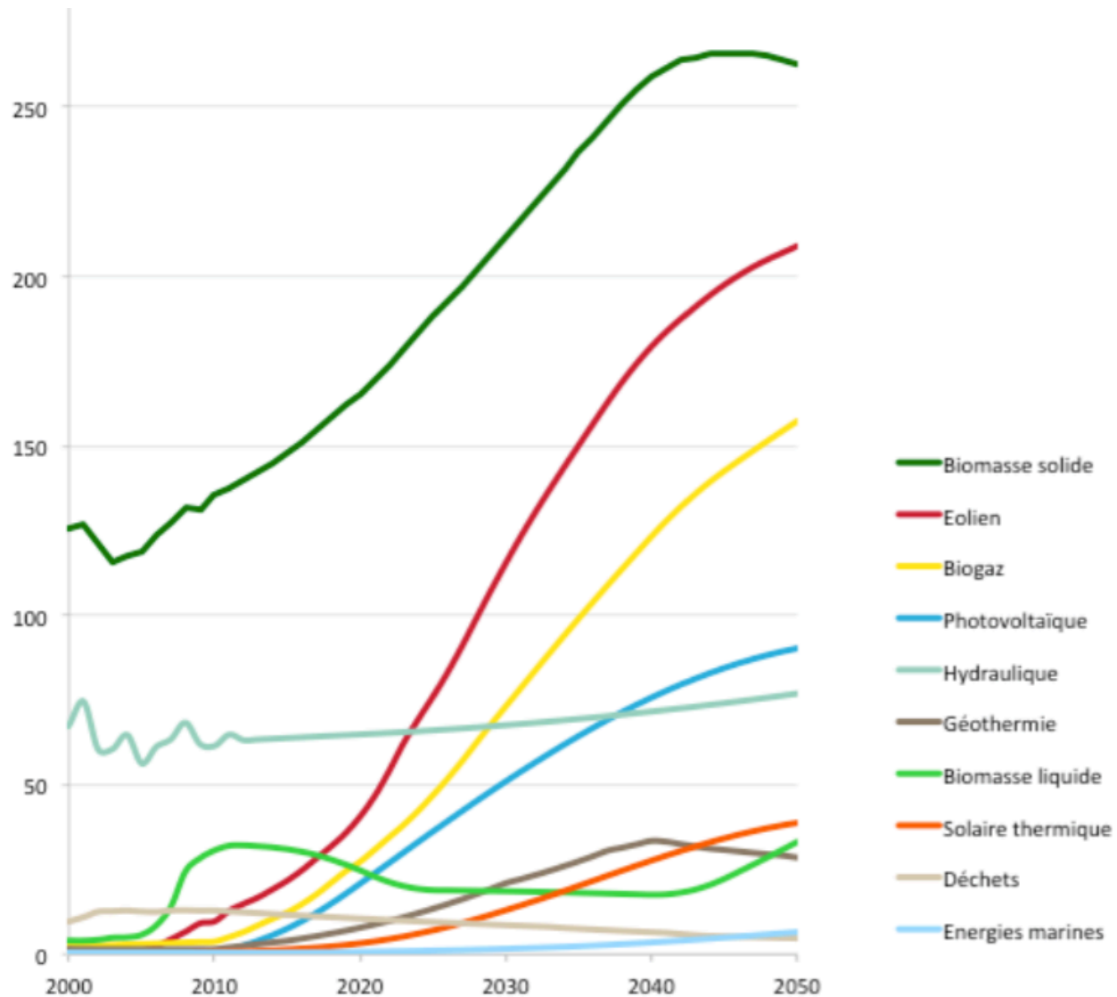
Figure 66 : Développement des différentes filières renouvelables dans le scénario négaWatt (en TWh)
